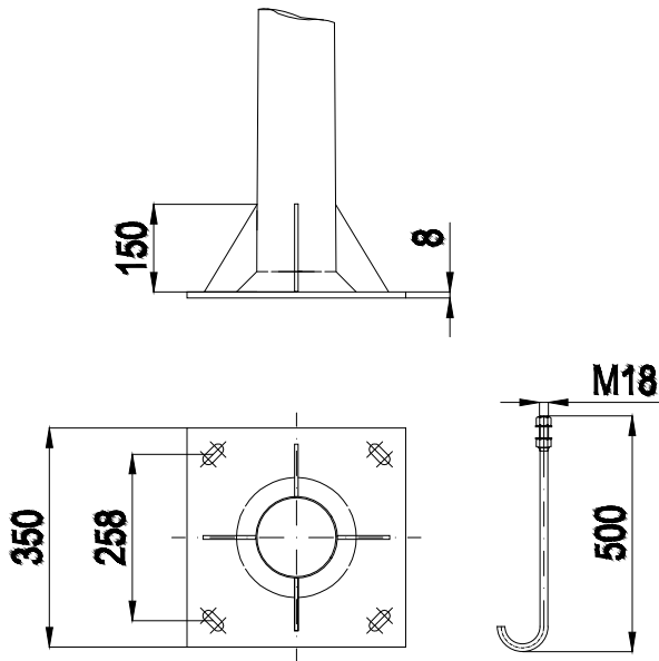
PLACA DE ASIENTO ALZADO
